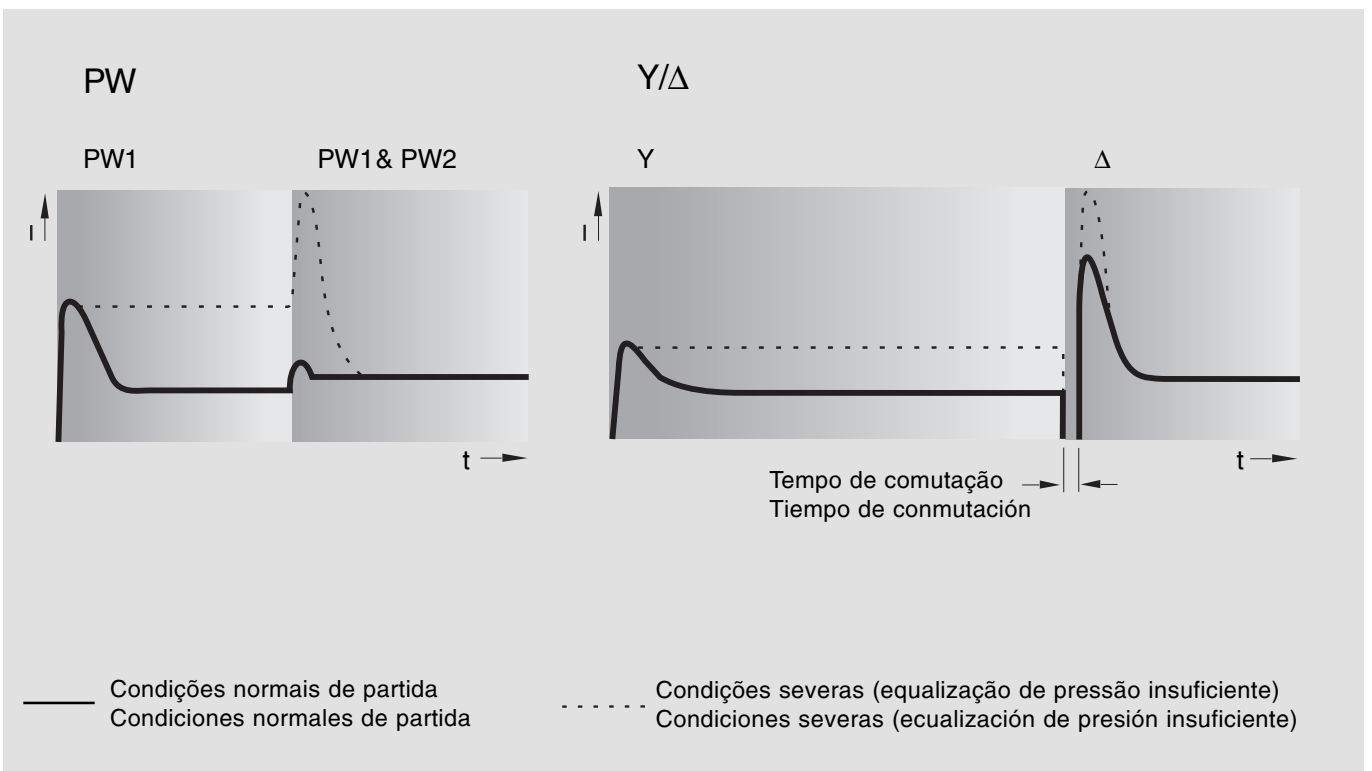
Fig. 2 – Características da corrente de partida PW1 Partida Dividida 1 PW2 Partida Dividida 2
