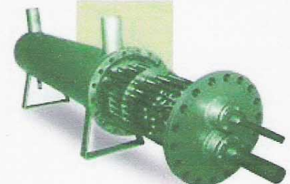
Evaporador aire forzado
