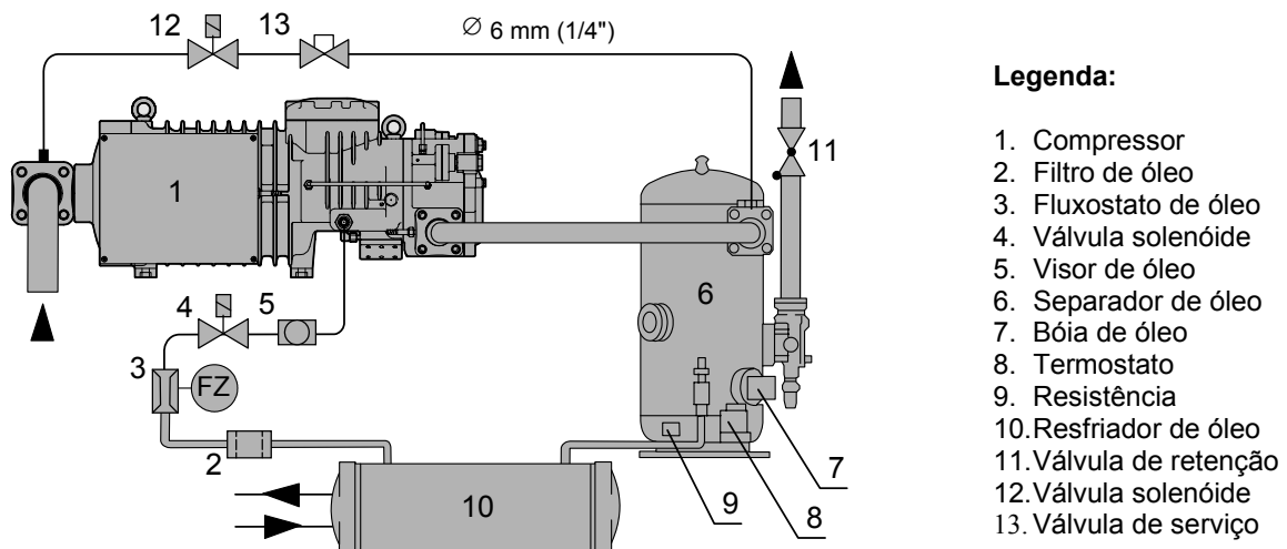
Diagrama 1 Circuito do óleo dos compressores parafuso da série OS..HS
